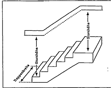
Nr. 2 gerade Treppe mit Unterzug
